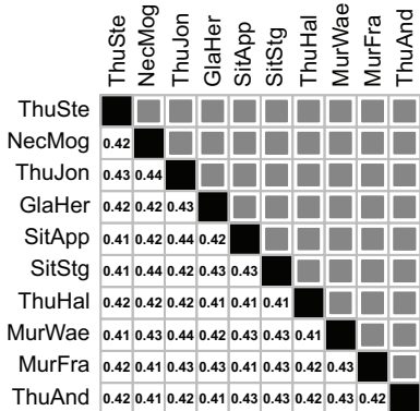
R-vine copula
