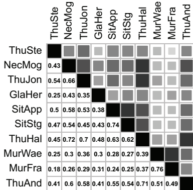
R-vine copula
